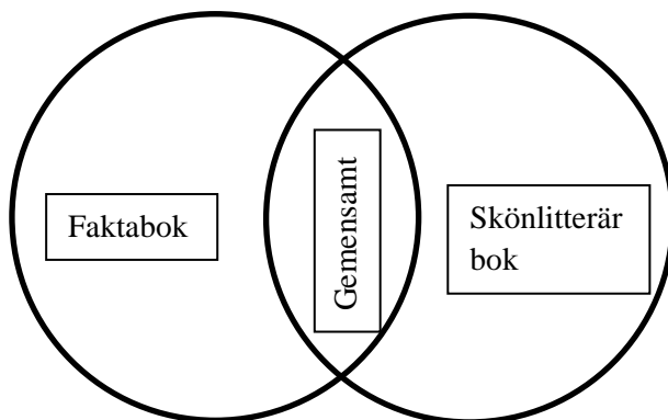
VENN-diagram
